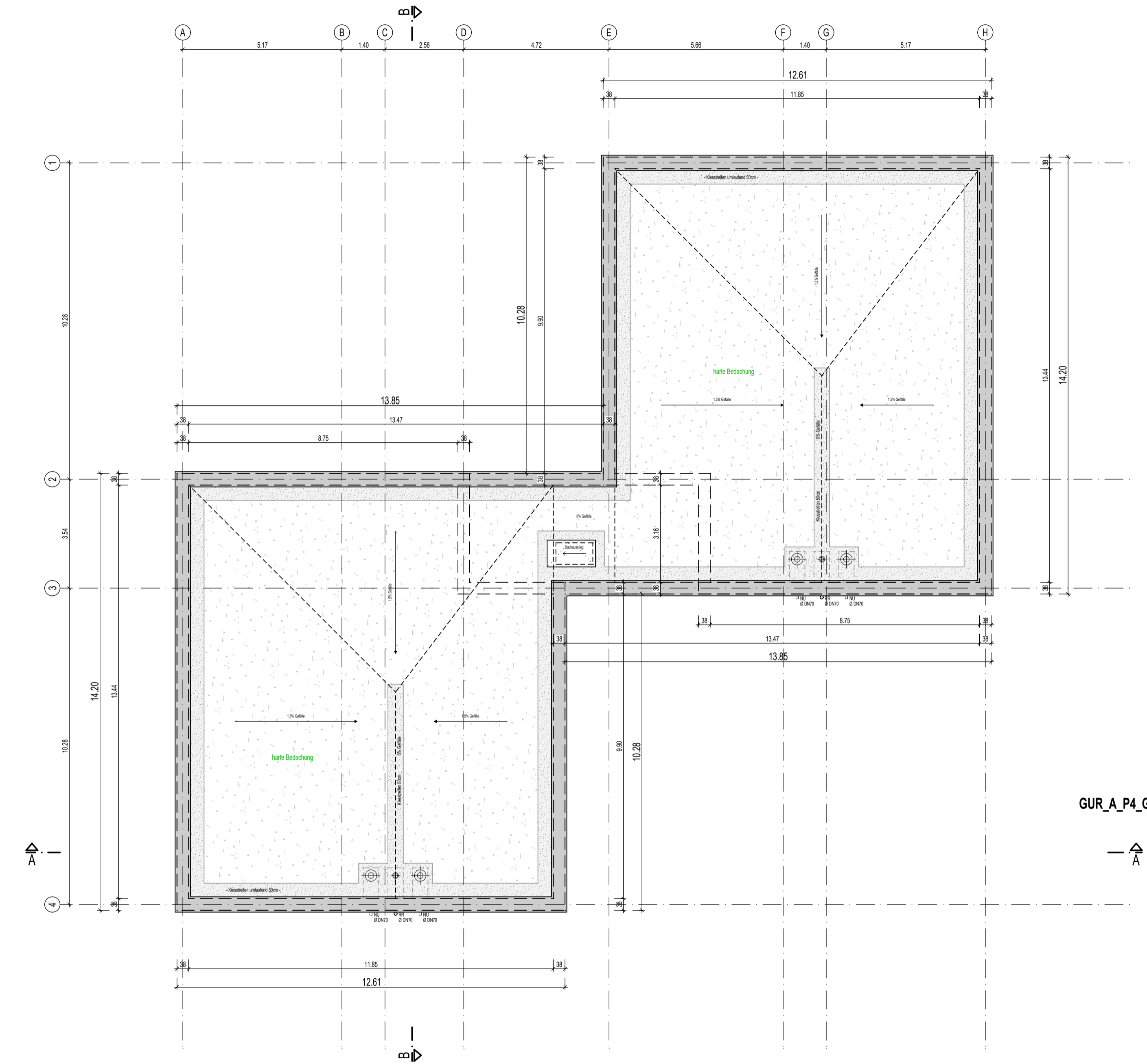
Dachaufsicht Haus 4 (+ Haus 5)
