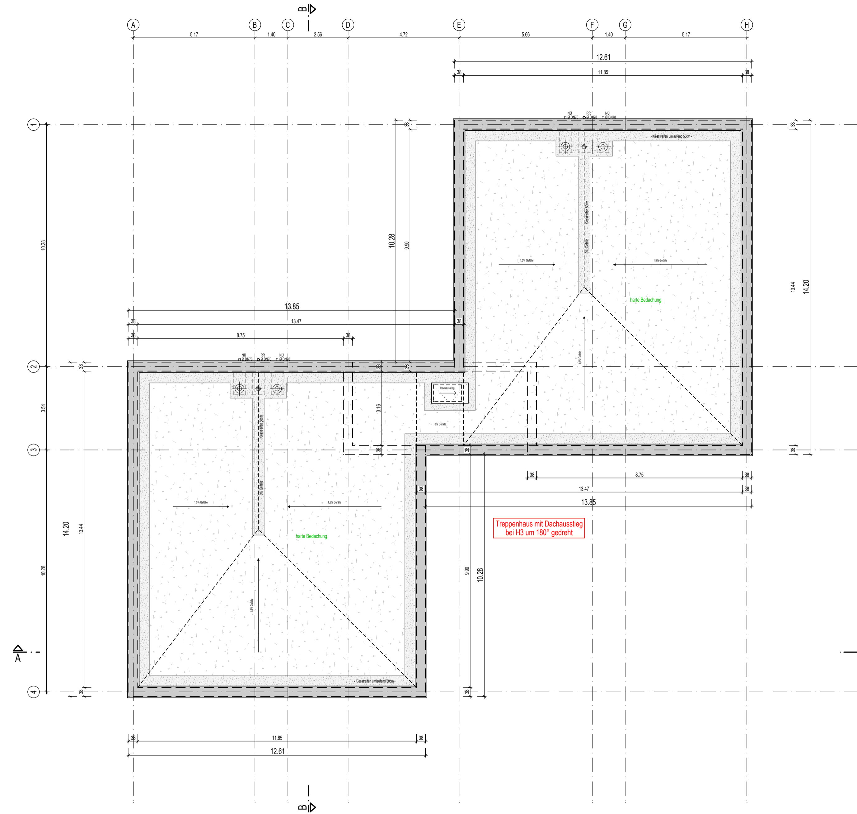
Dachaufsicht Haus 1 (- Haus 3)
