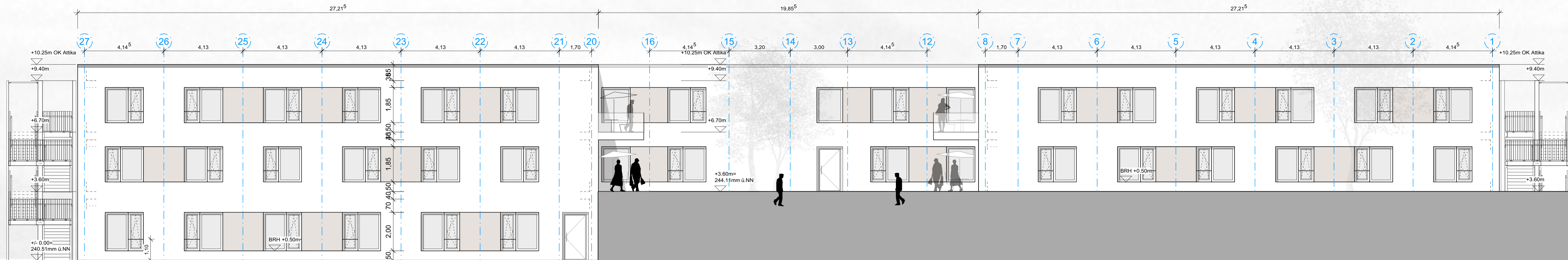
Ansicht Ost m: 1:100
