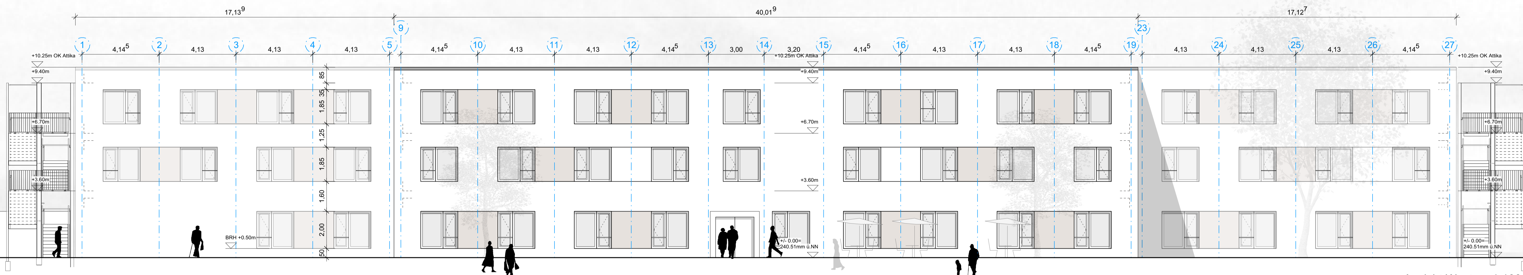
Ansicht West m: 1:100
